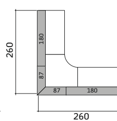
Eckkombination mit Verkettungsplatte
