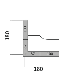
Eckkombination mit Winkelschreibtisch
