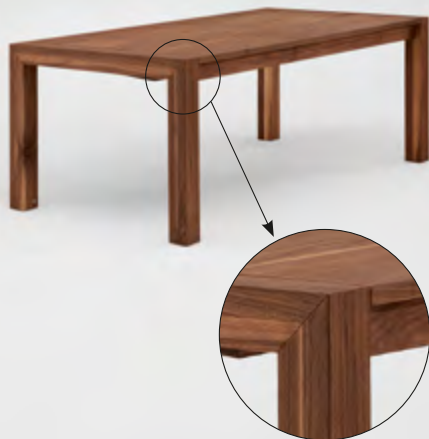
Tisch »FELIX« 4-Fuß Massivholztafeltisch mit Gehrungsgestell, Füße 9 x 9 cm. Höhe 77 cm.
